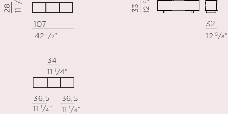
APO005 low table 107
